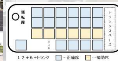
[観音開きトランク・モニター・手荷物スペース有] [Double doors trunk・monitor・Baggage space]
